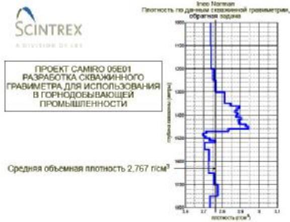
Рисунок 11: Место проведения испытаний в поселке Норман – Объемная плотность, патентованный алгоритм
