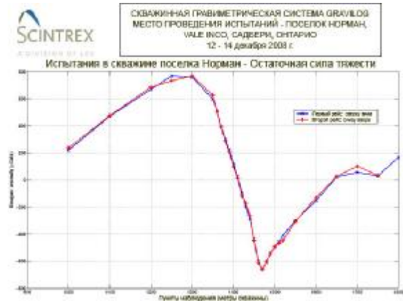
Рисунок 8: Место проведения испытаний в поселке Норман – Остаточная сила тяжести по результатам двух рейсов каротажного прибора
