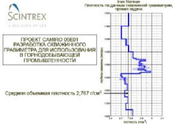
Рисунок 10: Место проведения испытаний в поселке Норман – Объемная плотность, обычный алгоритм
